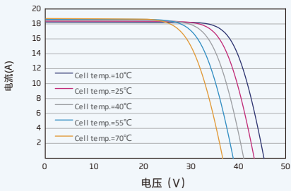
组件的I-V曲线 (665W)
