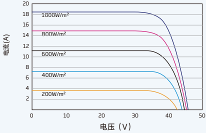
组件的P-V曲线 (665W)
